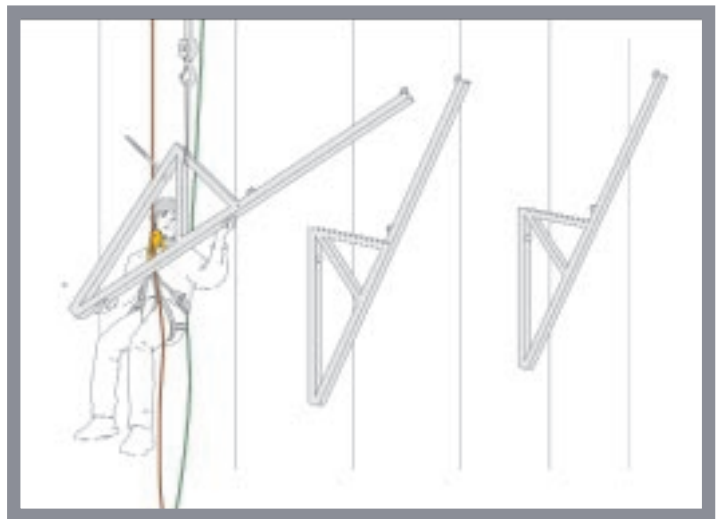
Accesso su corda per fissare i supporti di un impalcato
